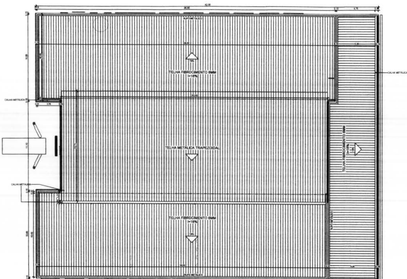
1 PLANTA DE LOCALIZAÇÃO E COBERTA Escala: 1 : 100
